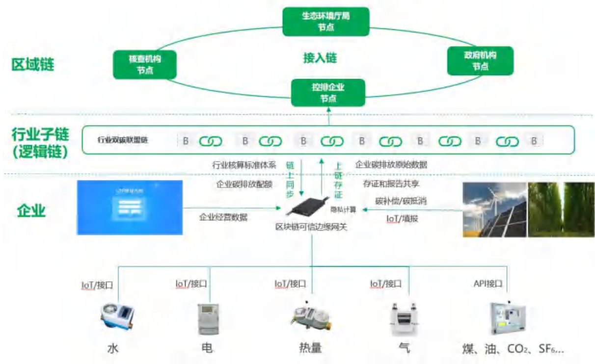
图 3.2.1 企业节点架构图
